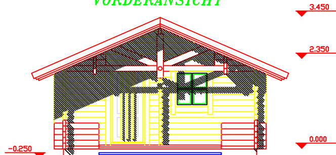
VORDERANSICHT
